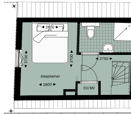
VERDIEPING 3
